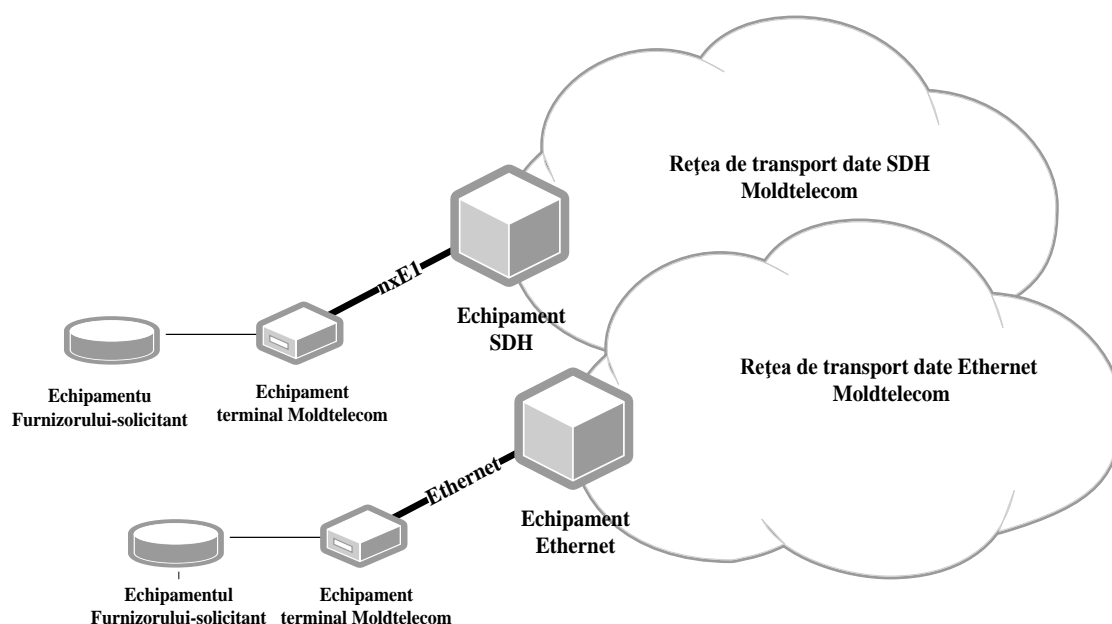
Fig. 2 Schema de organizare a serviciului de linii închiriate-segmente terminale
