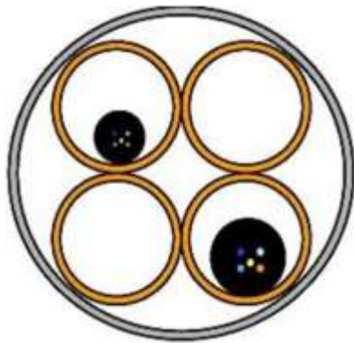
Fig. Nr. 4. Conductă principală cu 4 sub-conducte rigide
